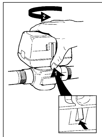
Fig. 3 Het plaatsen van de motor op de afsluiter
