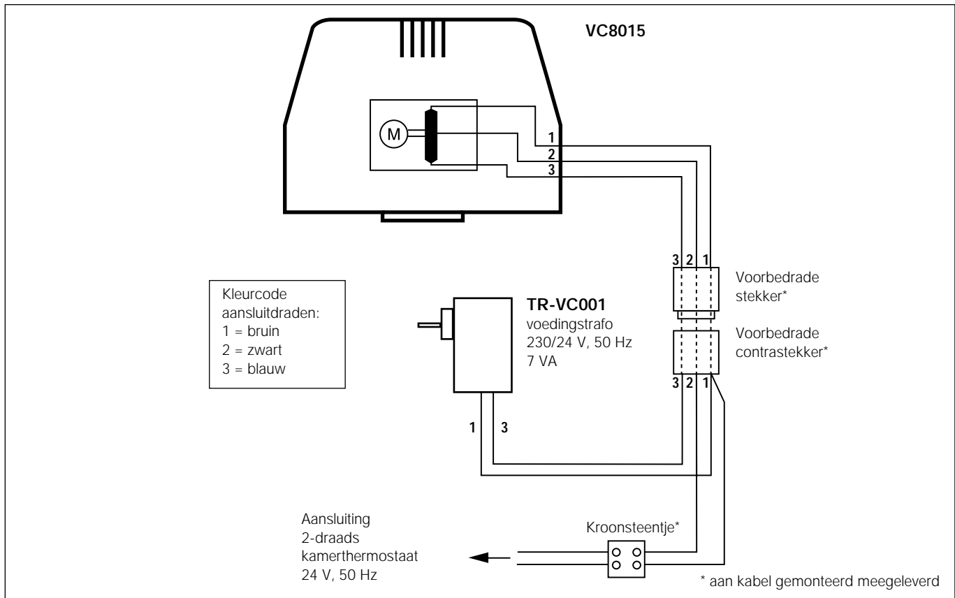
Fig. 5 Elektrische bedrading VC8015
