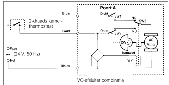
Fig. 6 Werkingsschema VC8015
